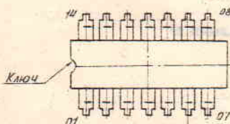
Схема расположения выводов *
